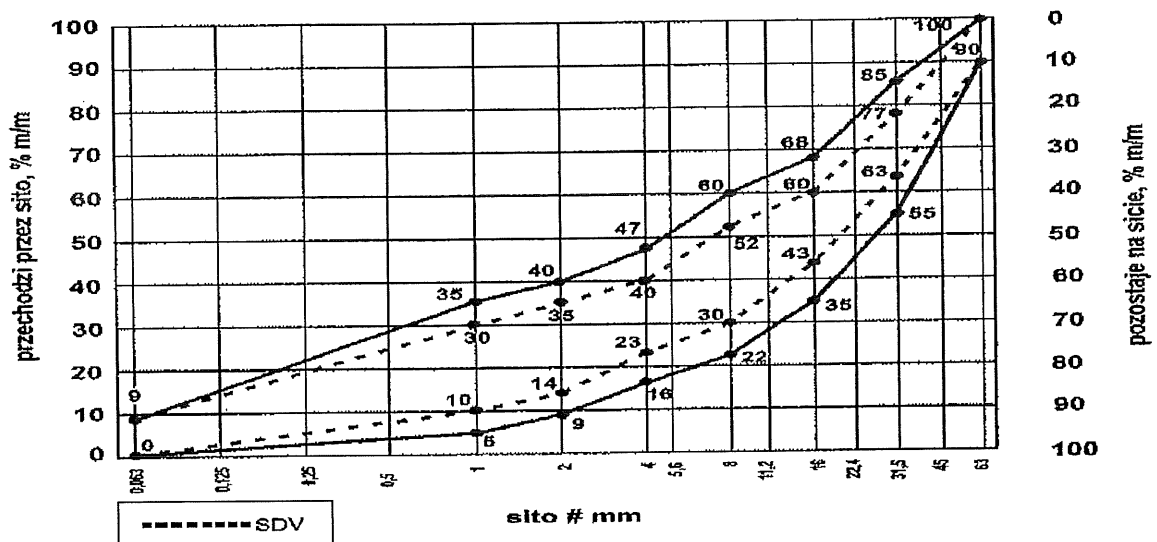
Rys. Krzywe graniczne uziarnienia mieszanki kruszywa niezwiązanego 0/63 mm do warstw podbudowy zasadniczej
